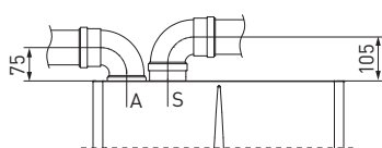
Rozdeľovacia sada Ø 80/80
