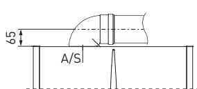
Koncentrická sada Ø 60/100
